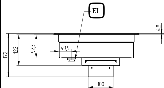
Oldalnézet
